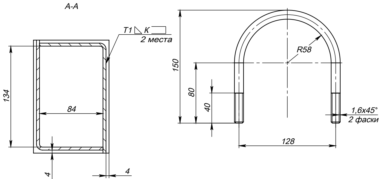
Поз.4 (Хомут)
